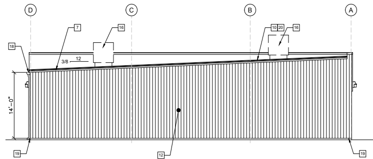
2 REAR ELEVATION A2 SCALE: 1/8" = 1'-0"
