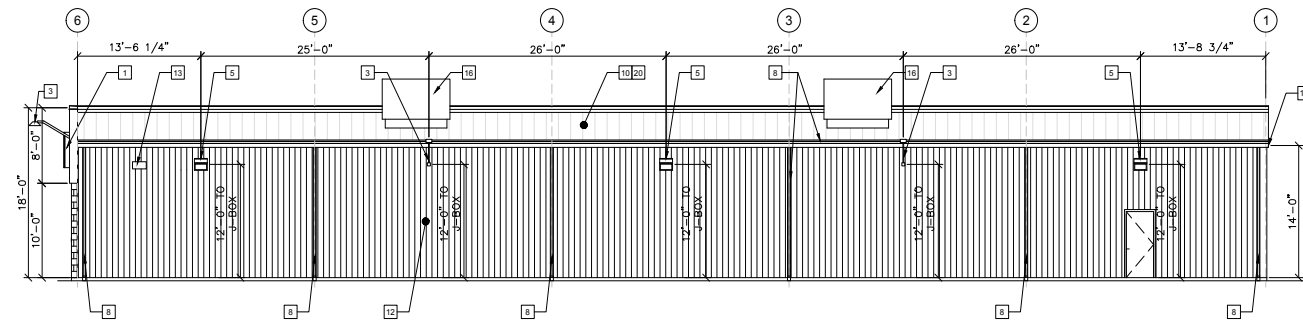
3 RIGHT ELEVATION A2 SCALE: 1/8" = 1'-0"
