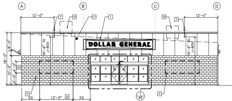
1 FRONT ELEVATION A2 SCALE: 1/8" = 1'-0"
